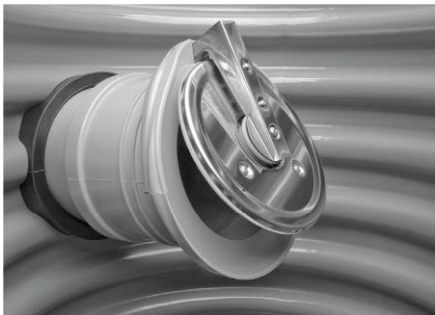
Egy példa a végszelep szerelésére Ø 110, akna mérete: Ø 315
